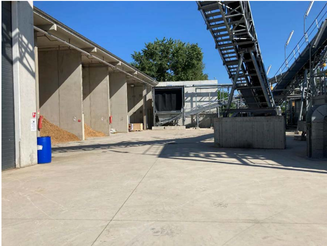
Figure 3 : alvéoles de stockage des intrants. Les mêmes alvéoles de stockage qu'avec ma biomasse seront utilisées pendant le projet pour stocker les CSR et bois B de façon distincte
